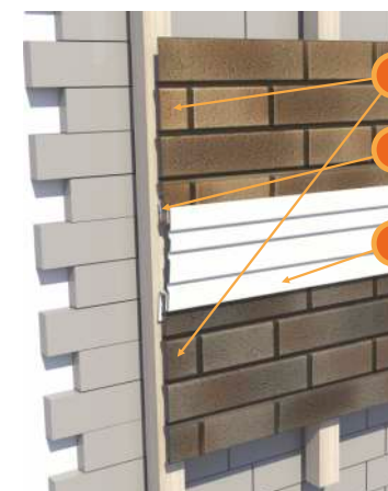
Межэтажный разделитель [ 120 мм ]
