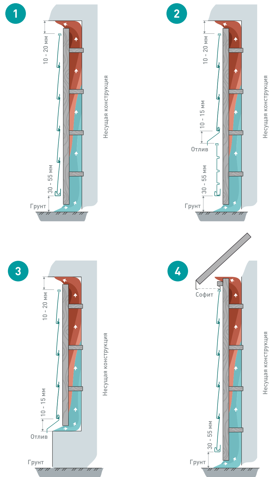
Варианты креплений навесного вентилируемого фасада с вариантами вентилируемых зазоров
